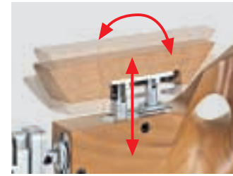
↑ Stufenlose Backenverstellmöglichkeit. Simple adjustments of cheek piece.
