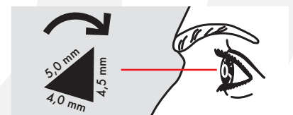
↑ Dreieckskorn für LP-@ ANSCHÜTZ. Triangular front sight for LP-@ ANSCHÜTZ. Best.-Nr.: 711.3710
