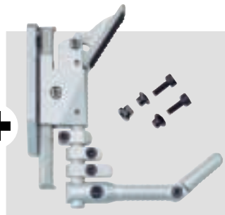
↑ Hakenkappe 2213-8700, kompl. mit Führungsplatte 2213-8510. Hook butt plate 2213-8700, complete with guide plate 2213-8510. Best.-Nr.: 700.3569
