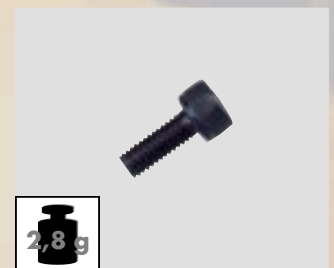
↑ Schraube für Füllstück , M5 x 10 DIN 912, ca. 2,8 g. Screw for filling piece , M5 x 10 DIN 912, approx. 2,8 g. Best.-Nr.: 007807
