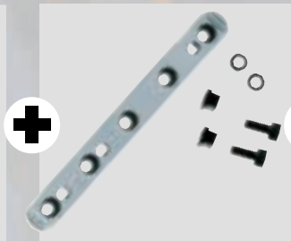
↑ Führungssäule 4759-4000 , 4760-20/1 mit Befestigungselementen. Guide column 4759-4000 , 4760-20/1 with fixing elements. Best.-Nr.: 700.3566
