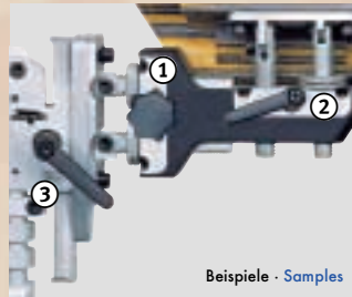
↑ Schnellklemmung, für Hakenkappe 4765 Fast clamp device, for hook butt plate 4765. Best.-Nr.: 700.3790 ③
