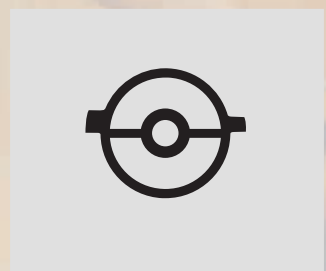
↑ Ringkorn 6522-9 , Ø 1,8; 2,0; 2,2; 2,4 bis 4,6 mm. Aperture insert 6522-9 , Ø 1.8; 2.0; 2.2; 2.4 to 4.6 mm. Best.-Nr.: 700.05xx
