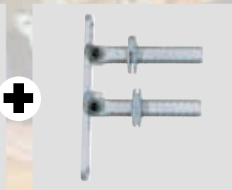
↑ Kappenausleger 4759-2000, 30 mm , mit schwenkbarer Säulenführung. Butt plate carrier 4759-2000, 30 mm , with tilting column guide. Best.-Nr.: 700.3564
