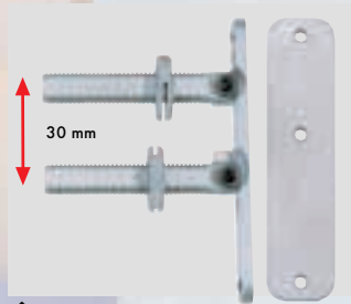
↑ Kappenausleger 4759-2000 , 30 mm mit schwenkbarer Säulenführung. Butt plate carrier 4759-2000 , 30 mm, with tilting column guide. Best.-Nr.: 700.3564
