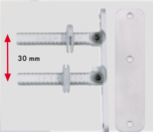
↑ Kappenausleger 4759-2000, 30 mm mit schwenkbarer Säulenführung. Hook plate carrier 4759-2000, 30 mm , with tilting column guide. Best.-Nr.: 700.3564
