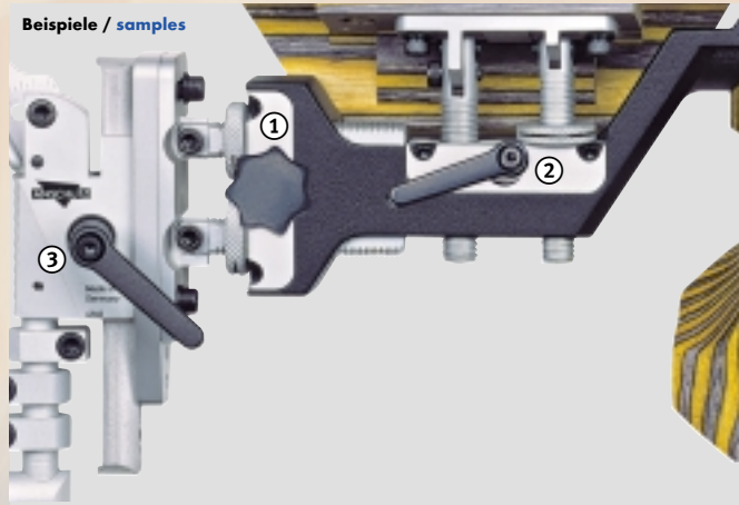
↑ Schnellklemmung, für neue Verstellung. Fast clamp device, for new adjustment. Best.-Nr.: 700.3780 ① Best.-Nr.: 700.3785 ② für Hakenkappe 4765 for hook butt plate 4765. Best.-Nr.: 700.3790 ③
