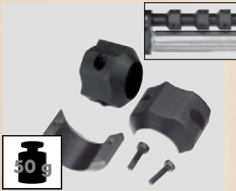
↑ Laufgewicht 4745 , 50 g, 2-teilig, Innen-Ø 20 mm. Two part barrel weight 4745 , 50 g, inner Ø 20 mm. Best.-Nr.: 700.6340
