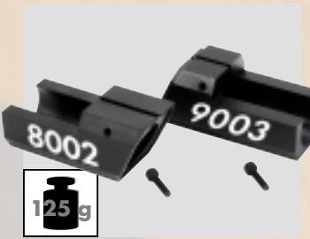
↑ Laufgewicht gross 8002/9003 , 125 g, Innen-Ø 20 mm. Barrel weight big 8002/9003 , 125 g, inner Ø 20 mm. Best.-Nr.: 700.6345 8002 Best.-Nr.: 700.6344 9003
