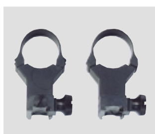
↑ Aufschubmontage 5525/26-1, 2-teilig, 31 mm hoch, mit Ring-Ø 26 mm. 2-piece mount 5525/26-1, 31 mm high, with rings Ø 26 mm. Best.-Nr.: 710.1610
