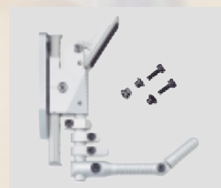
↑ Hakenkappe 2213-8700 , komplett mit Führungsplatte 2213-8510. Hook butt plate 2213-8700 , complete with guide plate 2213-8510. Best.-Nr.: 700.3569
