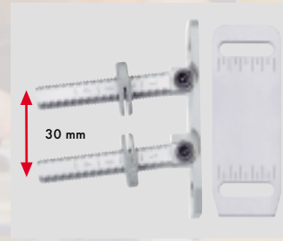
↑ Kappenausleger 2213-8300, 30 mm mit schwenkbarer Säulenführung für KK-Aluschäfte. Hook plate carrier 2213-8300 , with tilting column guide for small bore alu stocks. Best.-Nr.: 700.3563
