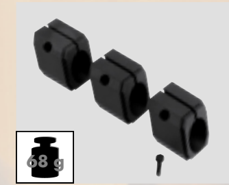
↑ Laufgewicht 4750 , 68 g, Innen-Ø 20 mm. Barrel weight 8002/9003 , 68 g, inner Ø 20 mm. Best.-Nr.: 700.6341
