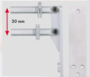
↑ Kappenausleger 9003/8002, 30 mm mit schwenkbarer Säulenführung. Hook plate carrier 9003/8002 , with tilting column guide. Best.-Nr.: 700.3573
