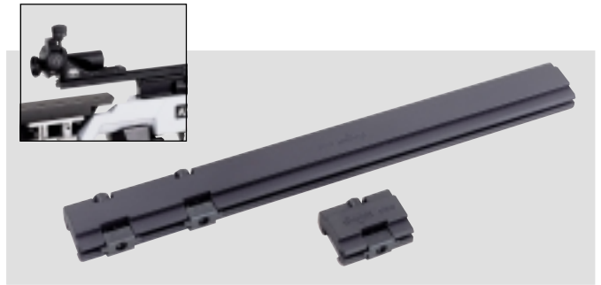
↑ Visierverlängerung für das Auflegeschiessen, 200 mm. Eine optimale Kombination aus Visierlinienverlängerung und -erhöhung, speziell für das Auflegeschiessen entwickelt. Der Blick durch die Visierung erfolgt durch den Auflageschützen grundlegend anders. Durch die Verlegung nach hinten und oben ist eine kompromisslose Anpassung an die unterschiedlichen Anschlagsarten möglich. Für Modelle ab 1907 und nachfolgende.
