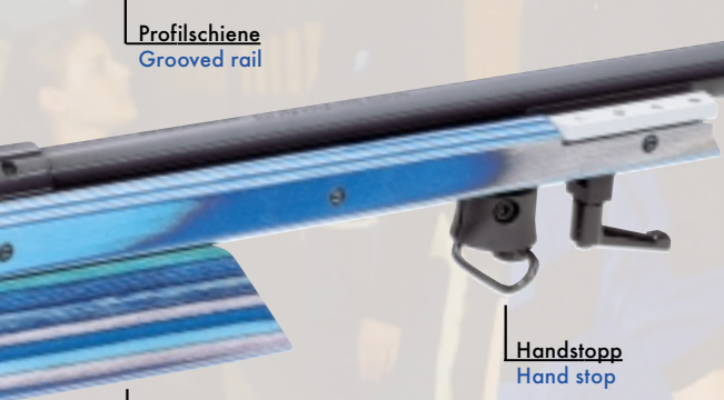
Vorderschafterhöhung Fore-end raiser block
